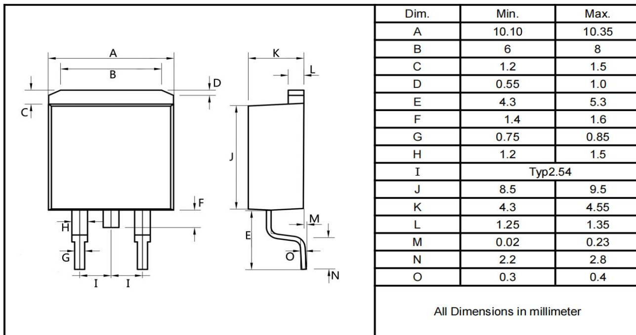
T0-263
